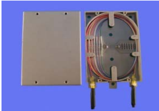
BAF-OCDB-A A 型收容盒
